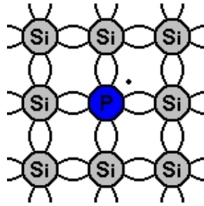
شکل ۲ بلور Si با ناخالصی نوع n
